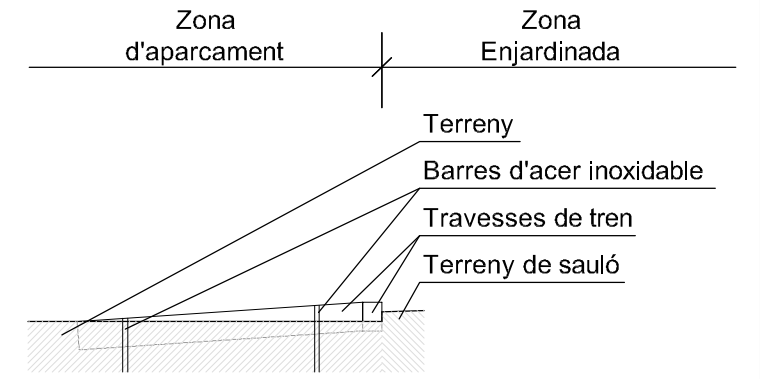
DETALL 1
