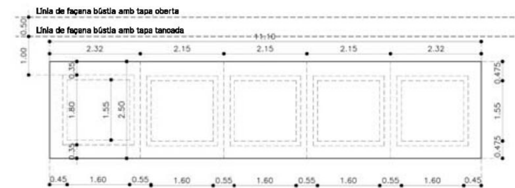
PLANTA TIPUS
