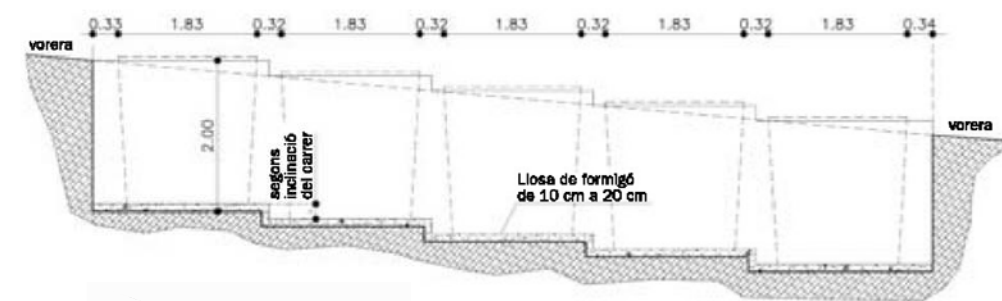
SECCIÓ TIPUS Colocació d'arquetes esgalonades o amb desnivell
