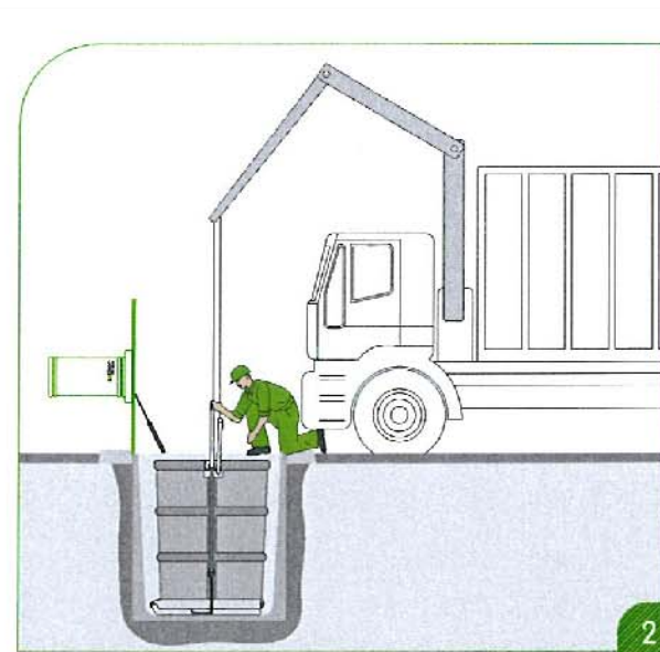
2 El operario acompaña las dos asas batientes para enganchar las argollas de las asas en los 2 ganchos de la pluma.
