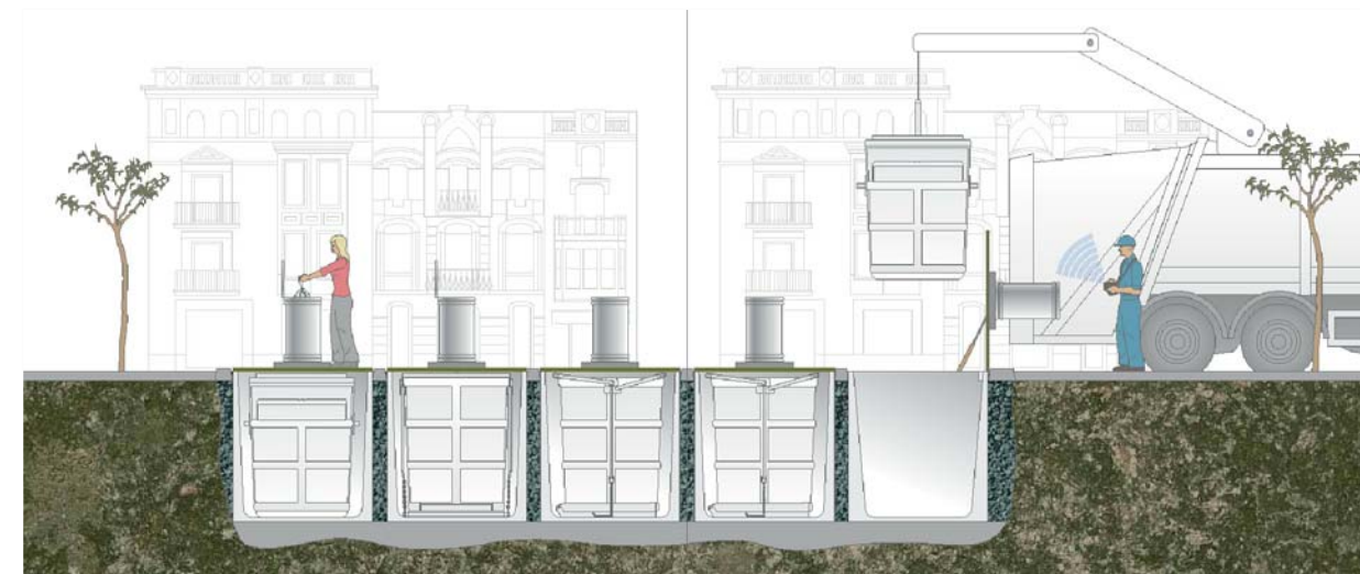
SECCIÓ TIPUS
